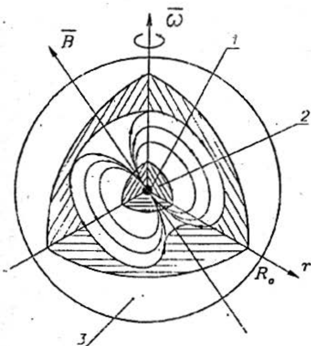
Рис. 1. "Устройство" шаровой молнии.
