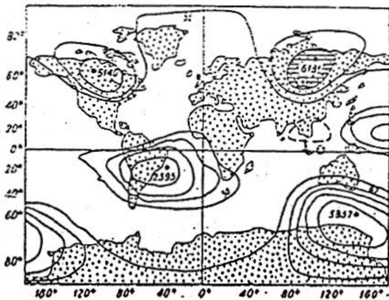
Рис. 2. Карта распределения модуля полного вектора ГМП эпохи 1965 г.
